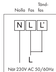
Inkoppling av självtest-armatur i permanentdrift.
