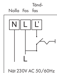
Inkoppling av självtest-armatur i permanentdrift med strömbrytarfunktion.
